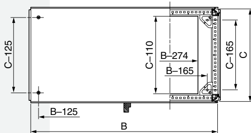
vnitřní rozměry – (dvojité dveře)
