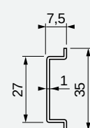
DIN lišta 35 mm typ B
