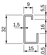
profil C
